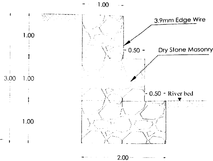
Sec A-A L=230M
